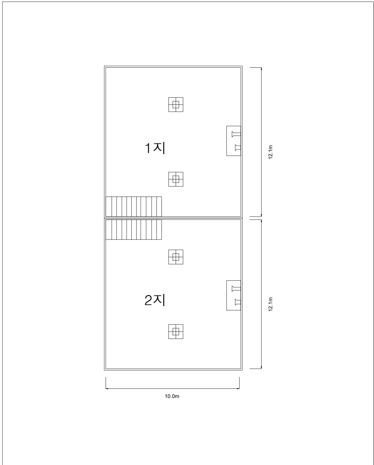
[그림 1.2-1] 남양5배수지(현대) 일반도
